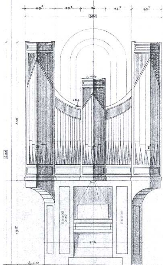
VORDERANSICHT
