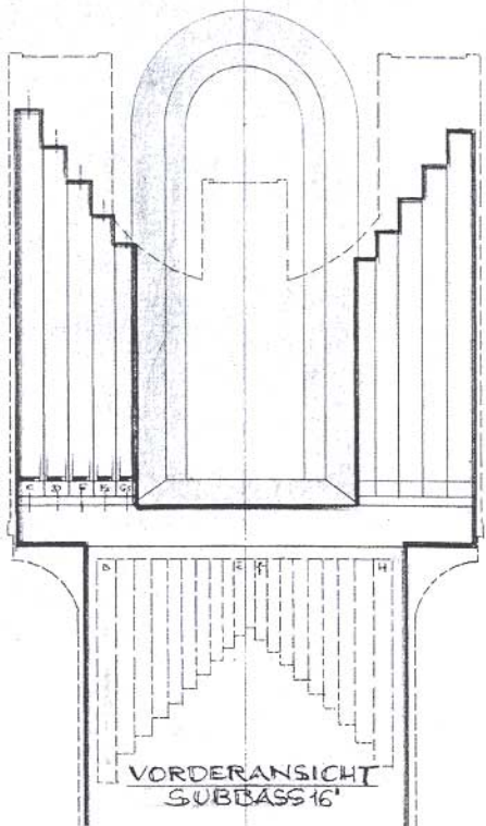
VORDERANSICHT
